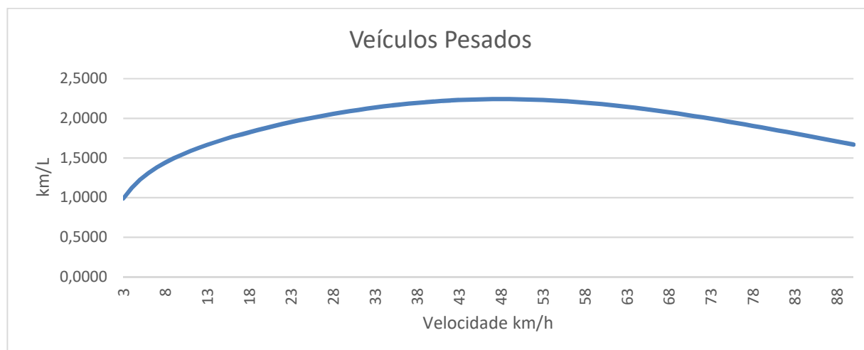
GRÁFICO 4.3 – GRÁFICO DO DESEMPENHO - CONSUMO DE COMBUSTÍVEIS PARA VEÍCULOS PESADOS
