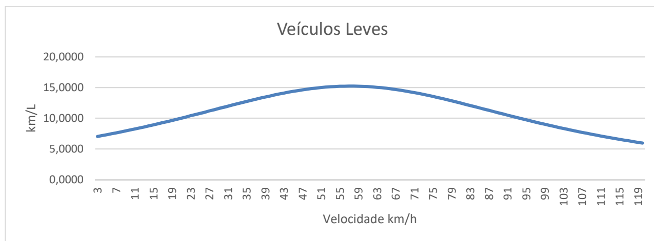
GRÁFICO 4.2 – GRÁFICO DO DESEMPENHO - CONSUMO DE COMBUSTÍVEIS PARA VEÍCULOS LEVES
