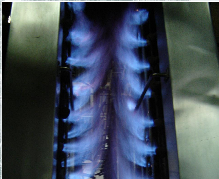
Chamuscador de suínos com Biogás
